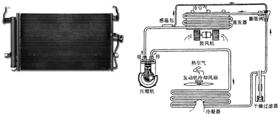
空調系統運作及冷凝器與蒸發器圖
