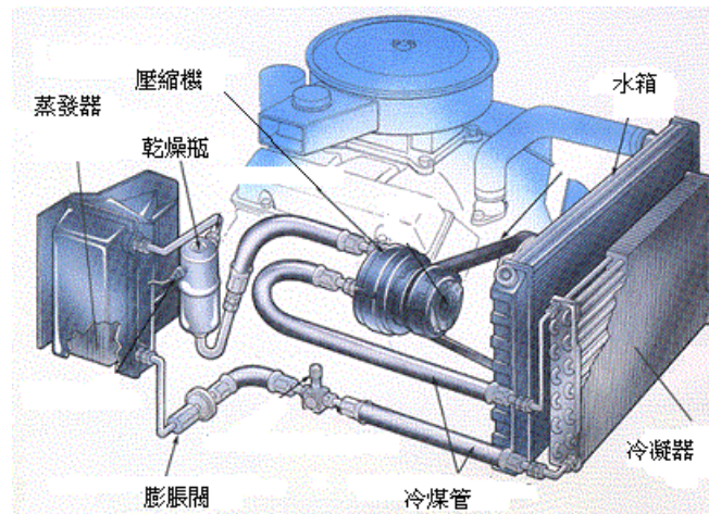
空調系統運作及冷凝器與蒸發器圖
