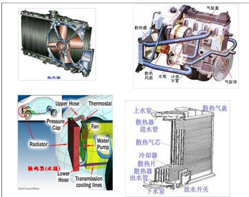
冷卻系統運作及水箱圖
